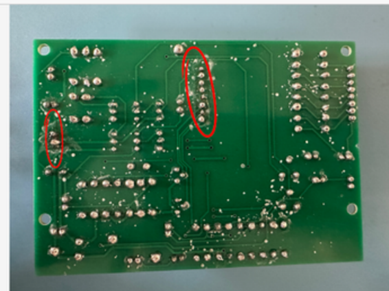
這些都是裝錯而導致電路板燒掉
