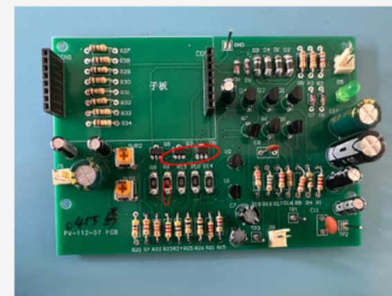
這些是當時沒焊好的地方
