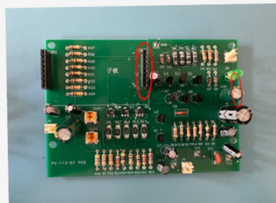
這些都是裝錯而導致電路板燒掉
